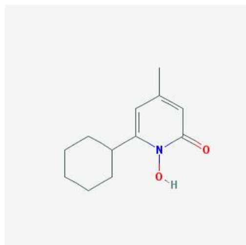
그림 1. 시클로피록스의 구조식
